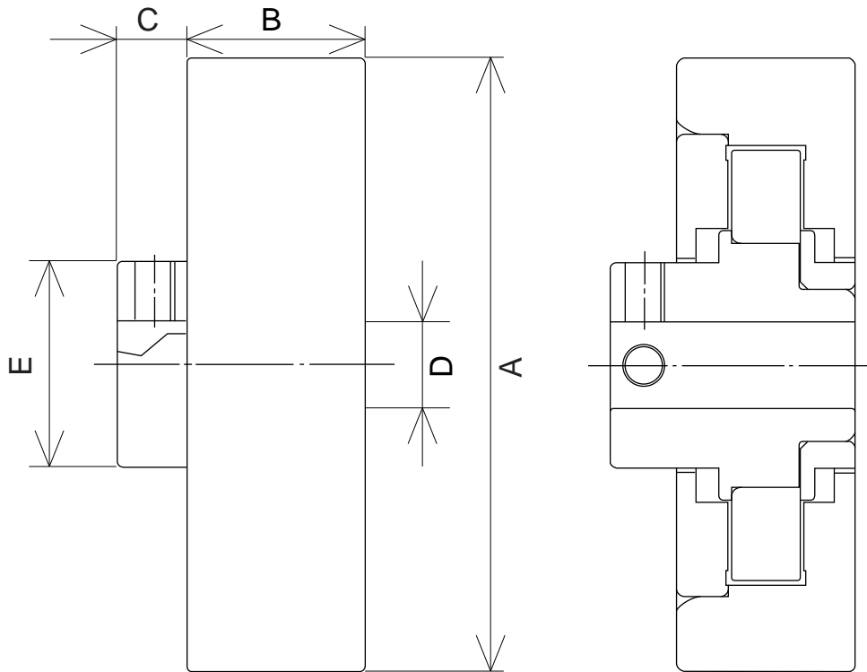
寸法図
